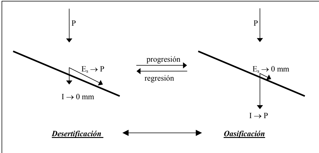
Figura 1. Oasificación contra desertificación. P = Precipitación; E_s = Escorrentía superficial; I = Infiltración
