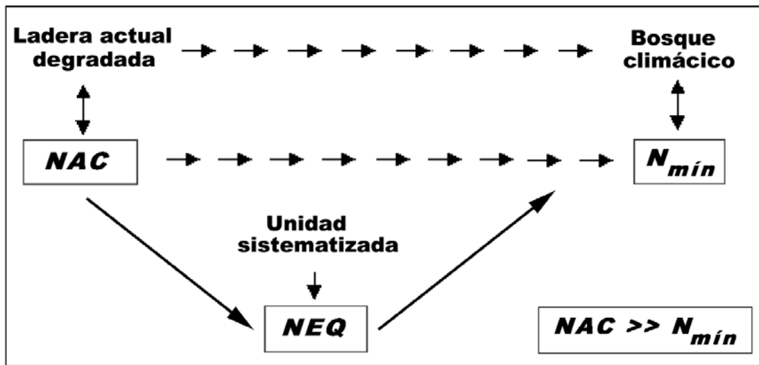
Figura 4. Serie progresiva del número de curva (MARTÍNEZ DE AZAGRA 1996). NAC = Número de curva de la ladera actual degradada; N_{mín} = Número de curva final en la ladera restaurada; NEQ = Número de curva equivalente de la unidad sistematizada.
