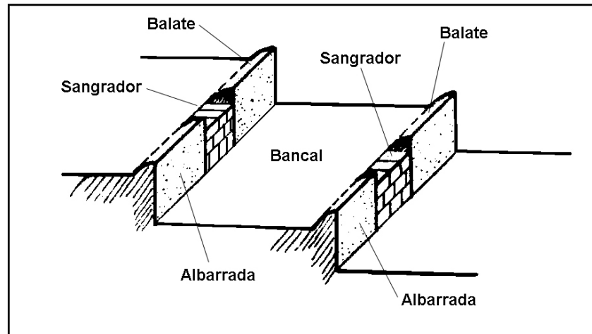
Figura 7. Riego a través de boqueras y sangradores (Fuente: MORALES 1969). Figure 7. Irrigation through 'boqueras & sangradores' (Source: MORALES 1969).
