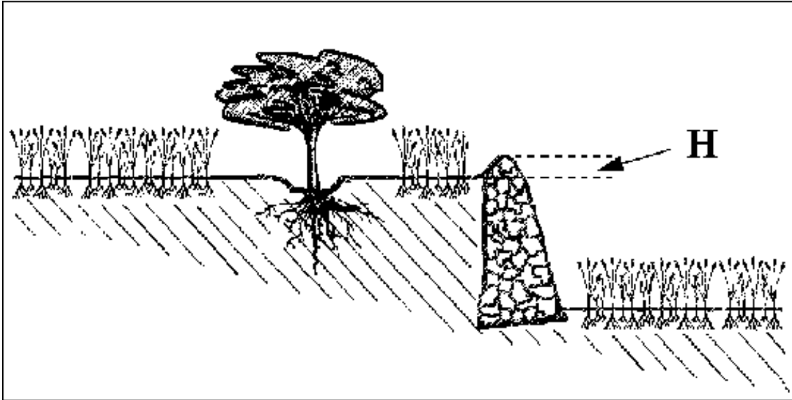
Figura 3. Bancal con su albarrada y su balate de altura H . Figure 3. Terrace with stone wall and ridge height ( H ).
