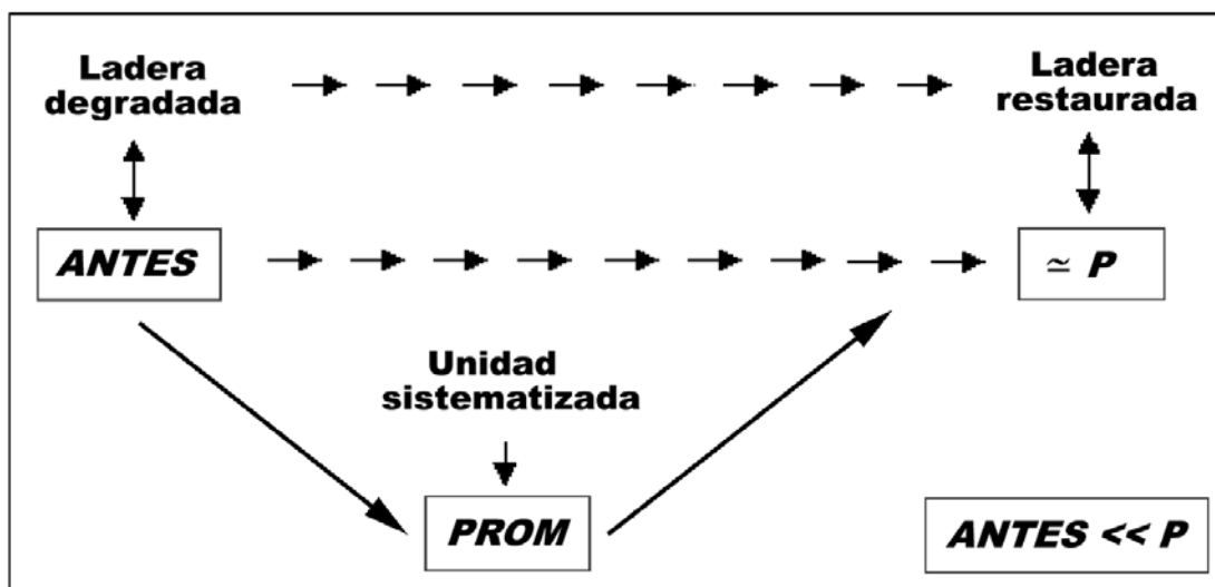
Figura 5. Sucesión progresiva de la infiltración y de las disponibilidades hídricas en una ladera degradada (MARTÍNEZ DE AZAGRA 1996). ANTES = Disponibilidad hídrica antes de la intervención, PROM = Disponibilidad hídrica promedio en las unidades sistematizadas, P = Precipitación
